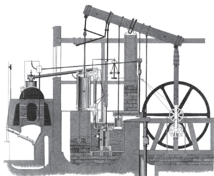
Парна машина Џејмса Вата
